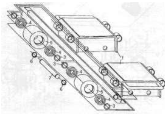
Устройство регулируемых платформ: СМ-60
